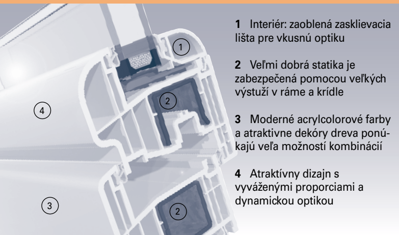
Detail štlpu
